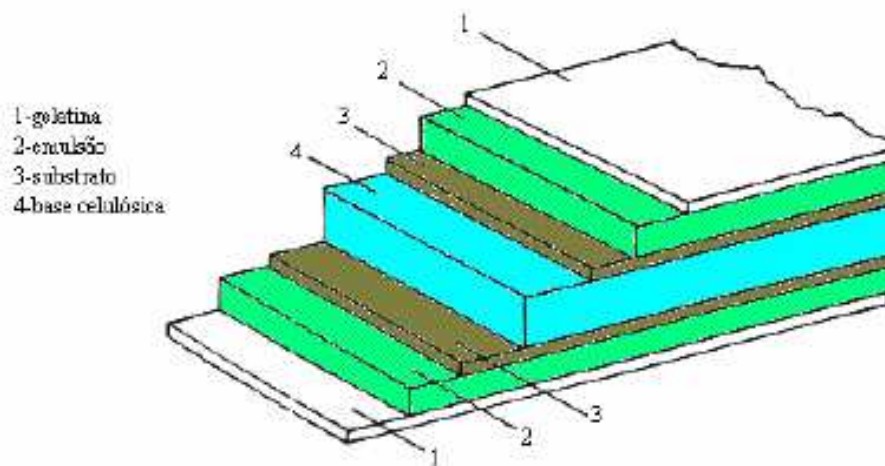
Figura 26 - Esquema de um Filme Radiográfico
