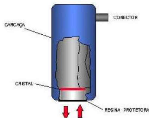
Figura 16 - Transdutor Normal ou Reto
