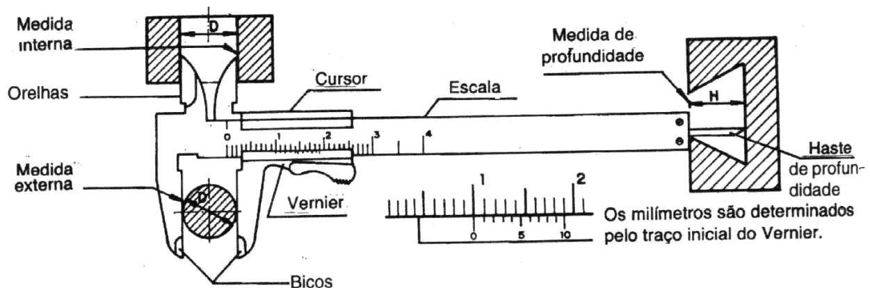
Figura 20 - Esquema Geral de um Paquímetro
