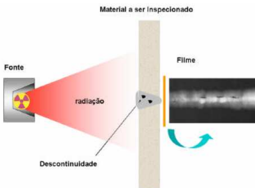
Figura 21 - Esquema Básico do Ensaio de Radiologia
