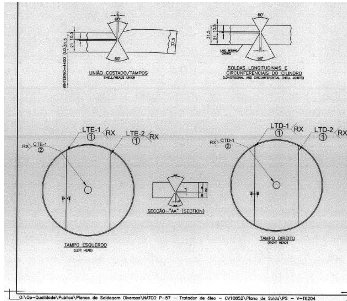
Figura 52 - Mapa de Solda 2 (Final)
