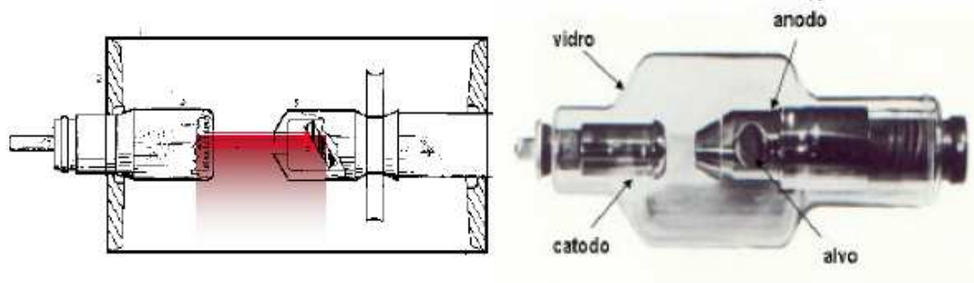
Figura 23 - Esquema Básico do tubo de Coolidge
