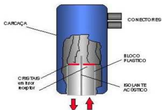
Figura 18 - Transdutor de Duplo Cristal
