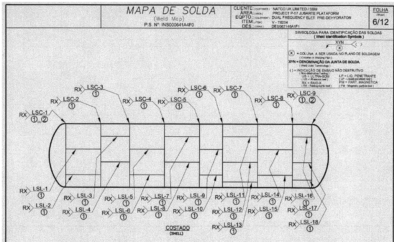
Figura 51 - Mapa de Solda 1
