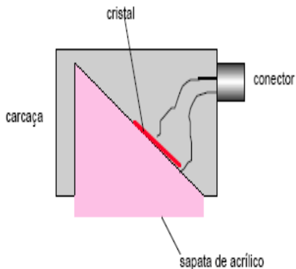
Figura 17 - Transdutor Angular
