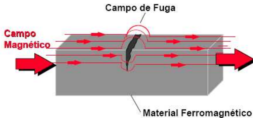
Figura 14 - Descontinuidade gerando um campo de fuga
