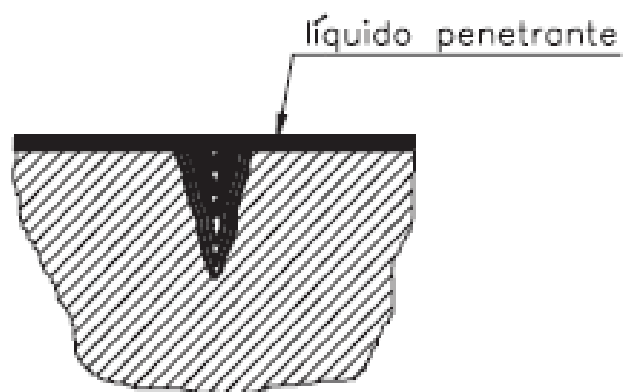
Figura 5 - Aplicação do Penetrante
