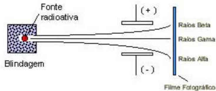
Figura 22 - Separação entre partículas alfa, beta e gama
