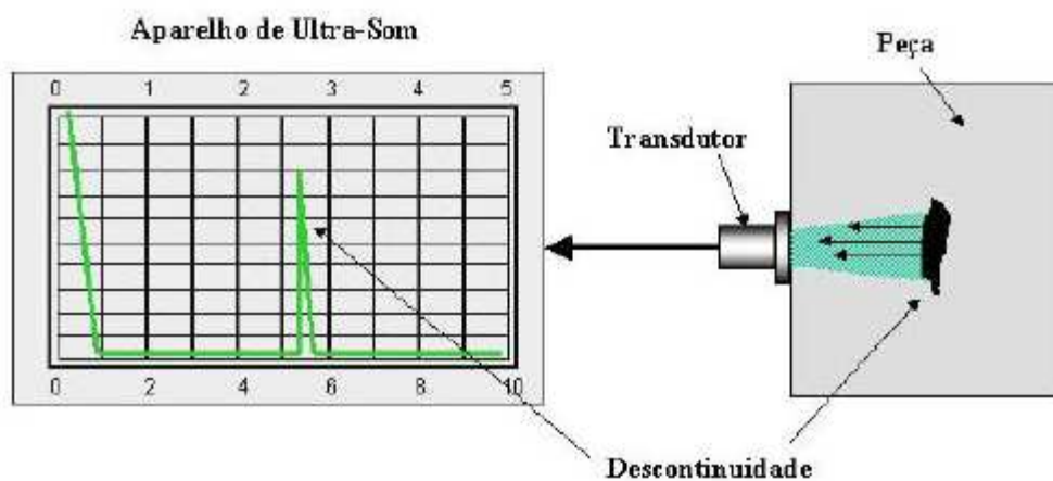
Figura 15 - Esquema básico do ensaio de Ultra-Som
